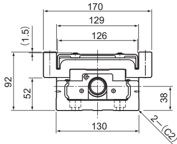
B-B横断面
