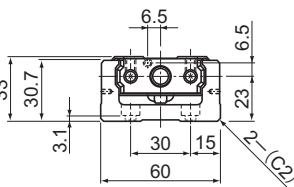
B-B横断面
