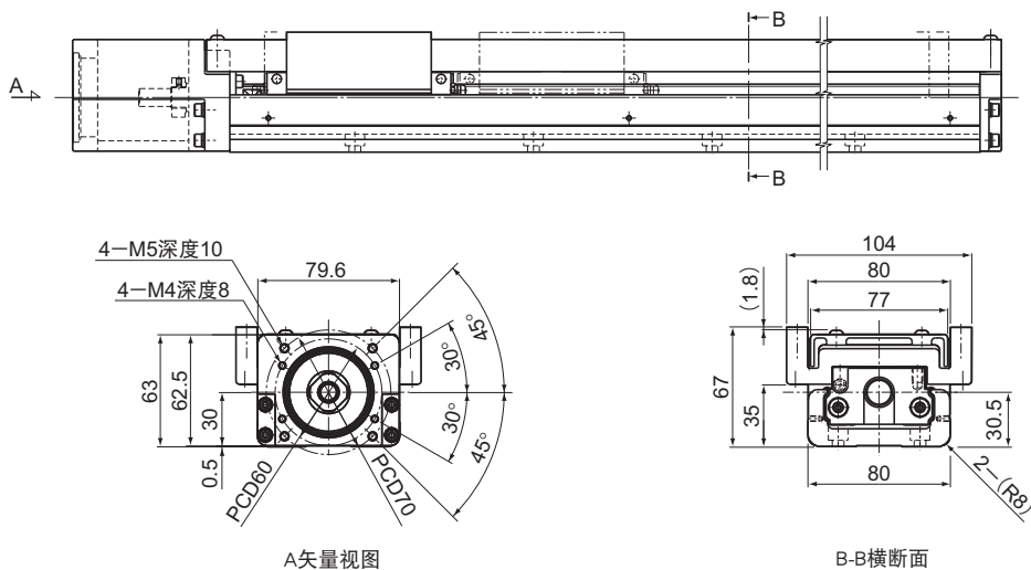
A-A矢视图
