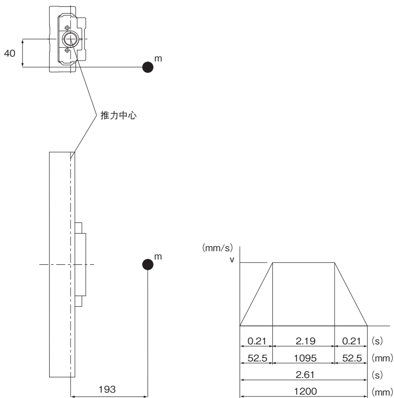
图2 速度线图
