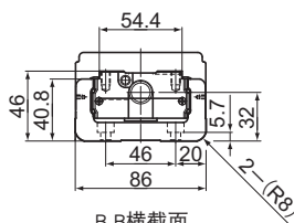
B-B横截面
