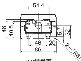
B-B横截面
