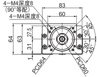
A-A 矢量视图
