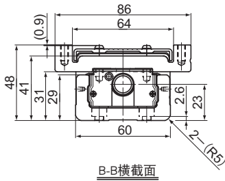
B-B横截面
