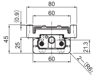
B-B横断面
