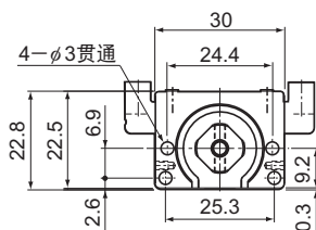
A-A视图
