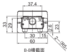
B-B横截面
