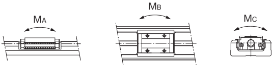
长型螺母滑块1个 (SKR-A型)
